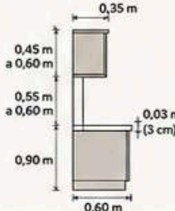
VISTA LATERAL (CORTE)
