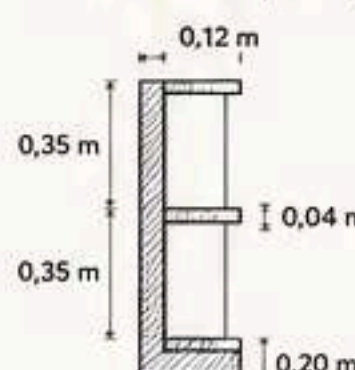
VISTA LATERAL (CORTE)
